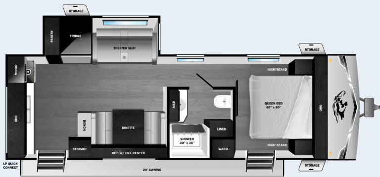
230MKD OPTIONS A, C & D
